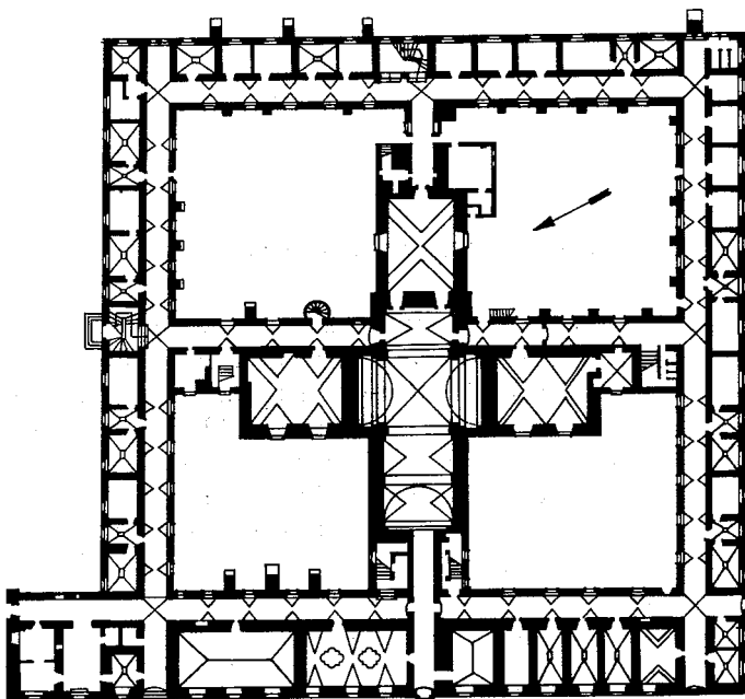
Rzut przyziemia klasztoru i kościoła wg pomiarów z 1965 r.
