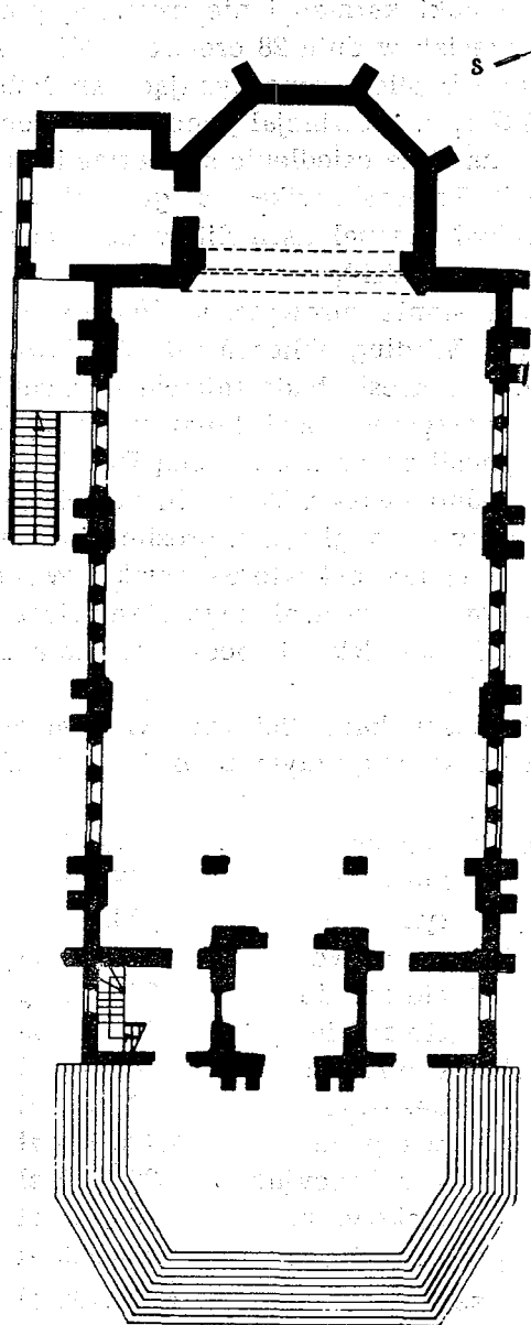
17. Łódź. Rzut przyziemia kościoła Św. Józefa wg pomiarów z 1968 r.
