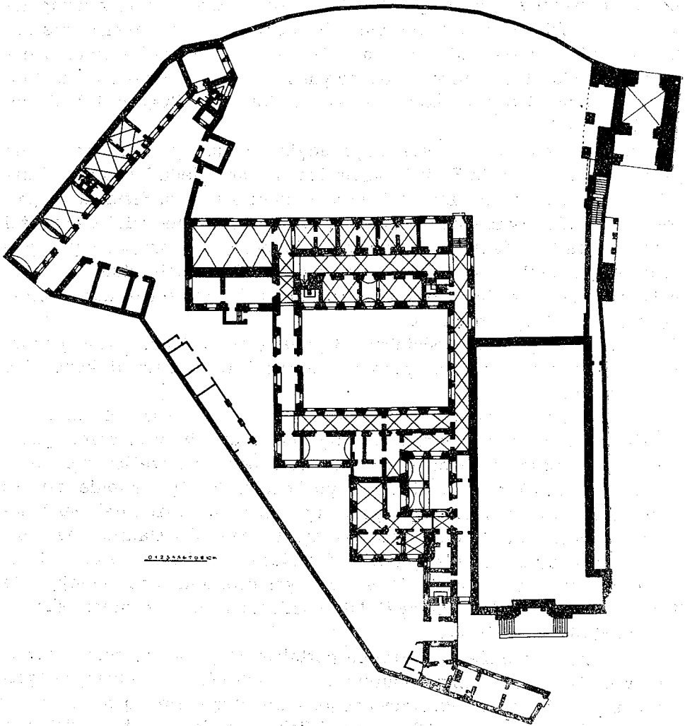
12. Wilno. Rzut przyziemia klasztoru i kościoła Św. Teresy wg pomiarów z 1930 r.
