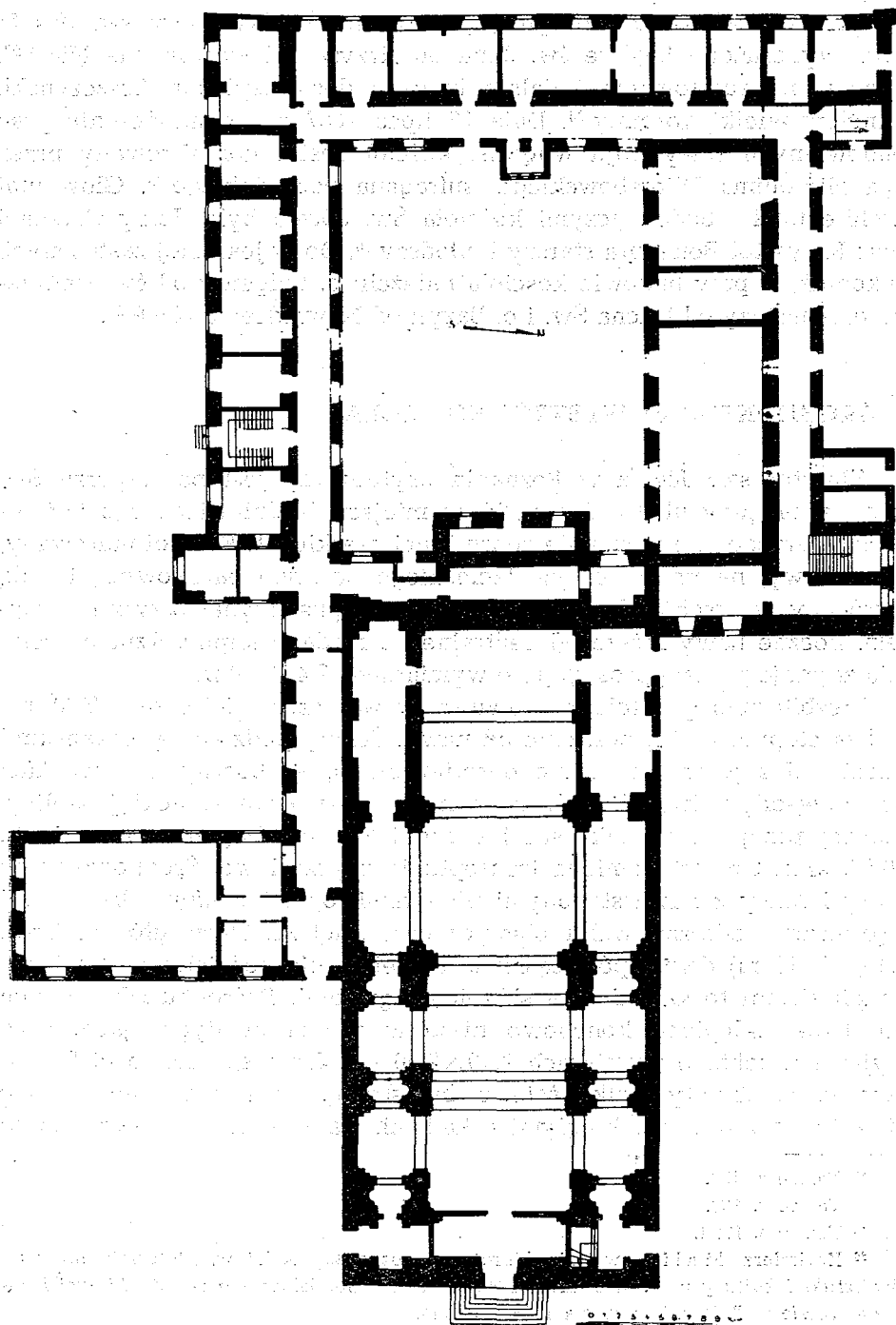
10. Poznań. Rzut poziomy kościoła i klasztoru Św. Józefa
